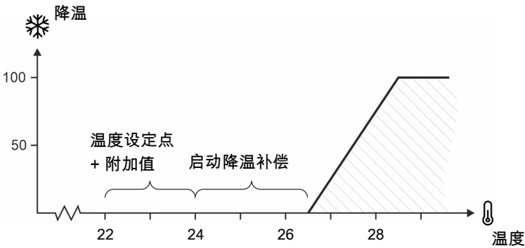
图 26: 降温 启动降温的前提条件是，通风被设置为 最大通风量 ，或者室外温度高于 温度设定值 。
