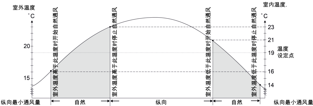
图 21：自然通风是否启动取决于当前的室外温度。温度设定点为 19°C。
