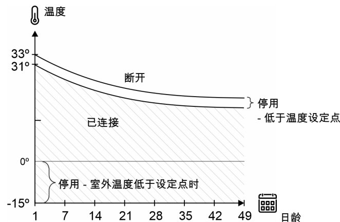
图 17: 热回收装置 - 室外高低温限定
