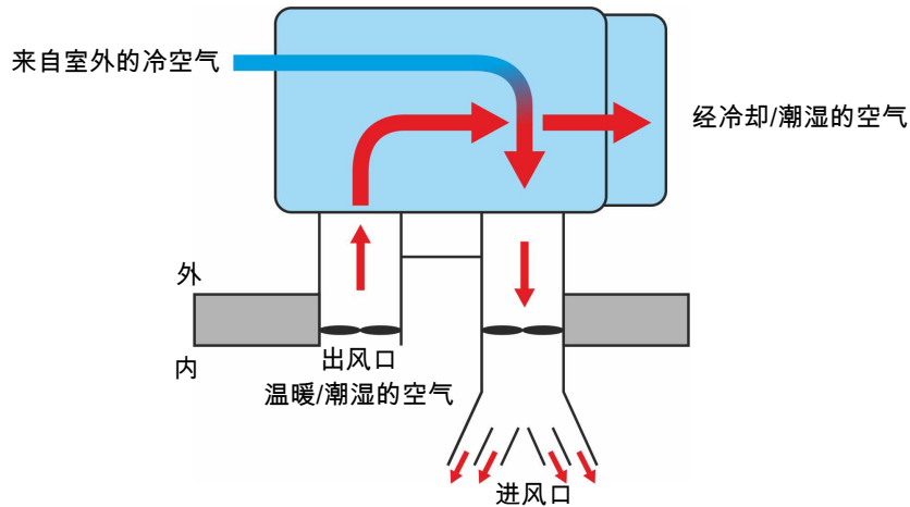
图 16: 热回收装置原理的示例。
