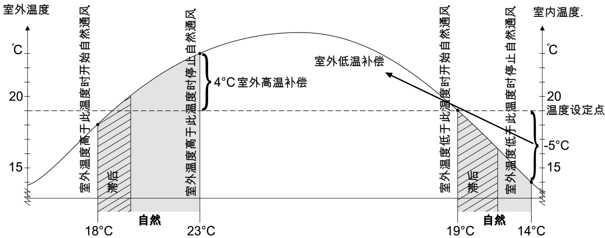
图 22：自然通风是否启动取决于当前的室外温度。
