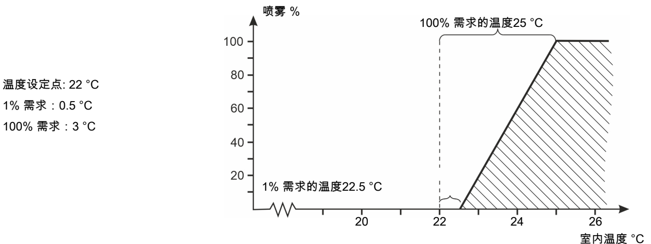
图 29: 根据室内温度喷雾
