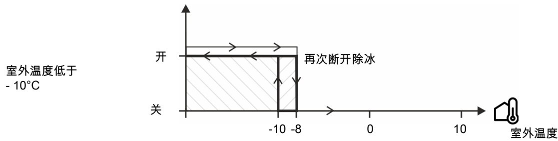
图 15: 启动除冰功能
