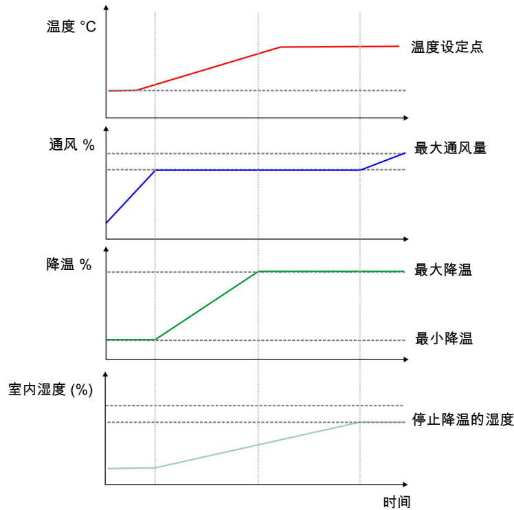
图 27: 为了维持所需的室内温度, 在通风水平达到最大通风量之前开始降温。当降温无法维持温度时, 再次增加通风量。
