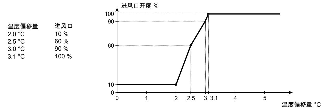
图 10: 综合扩散进风口 - 无级进风口根据室内外温度打开
