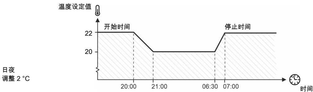
图 7: 日夜调整设置为夜间温度降低。
