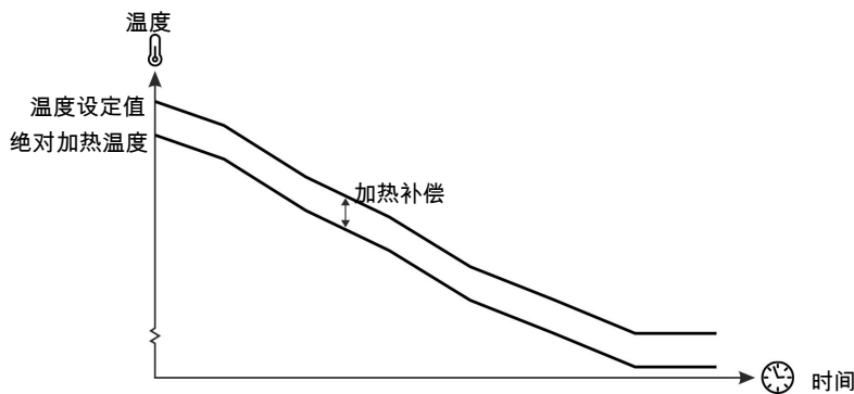
图 33: 设置加热补偿
