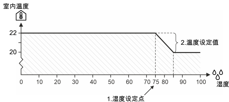
图 14: 温度下降控制湿度
