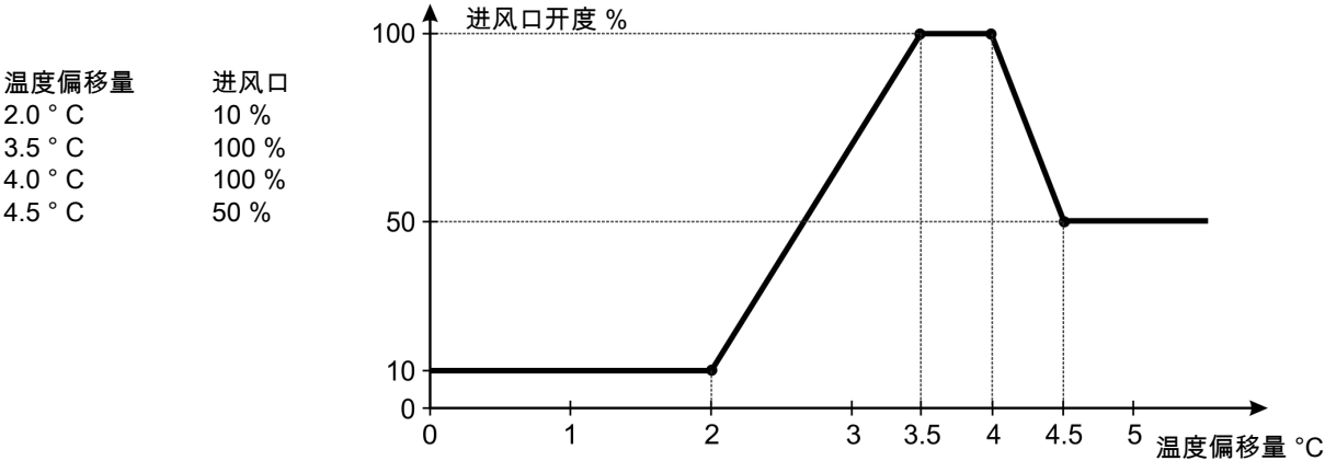
图 9: 综合扩散进风口 - 在室外温度较高时减小无级进风口的开度
