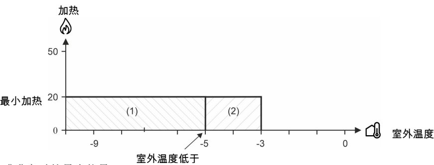
图 35: 室外温度降低或升高时的最小热量
