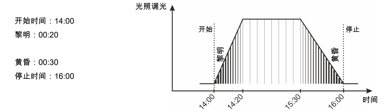
图 39：正常调光 黎明和黄昏被纳入照明时段。
