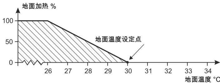
图 36: 带温度传感器的地面加热
