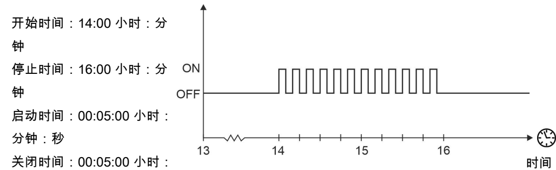
图 24: 24 小时时钟控制
