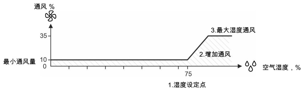
图 13: 湿度通风: 1. 空气湿度超过湿度设定点。2. 控制器增加通风量。3. 增加到最大的湿度通风 (35%)。
