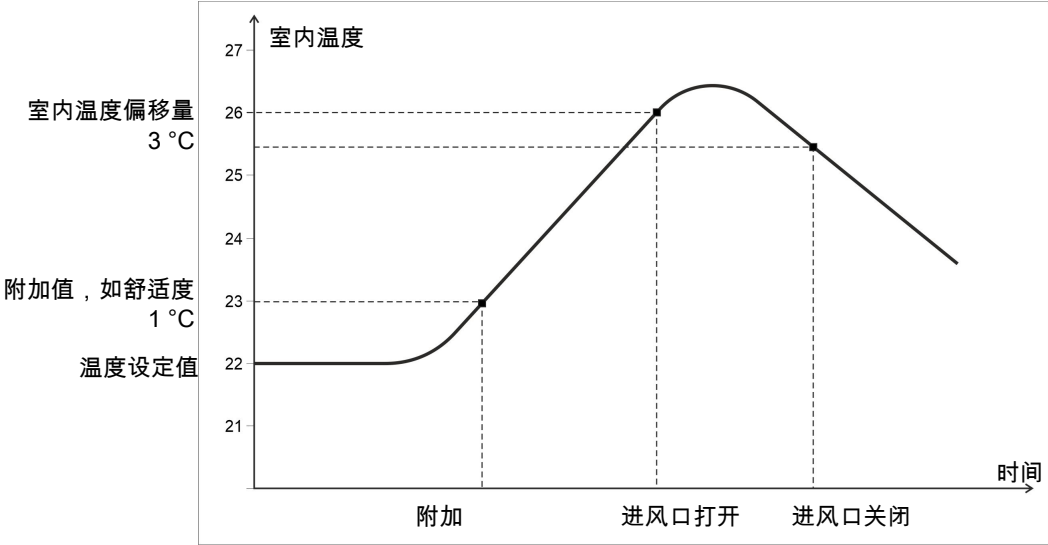
图 8: 综合扩散进风口 - 室内温度调节
