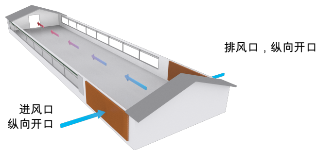
图 20：自然通风与纵向通风结合使用的房舍示例，纵向通风。
