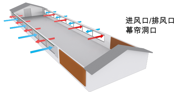
图 19：自然通风与纵向通风结合使用的房舍示例，自然通风。
