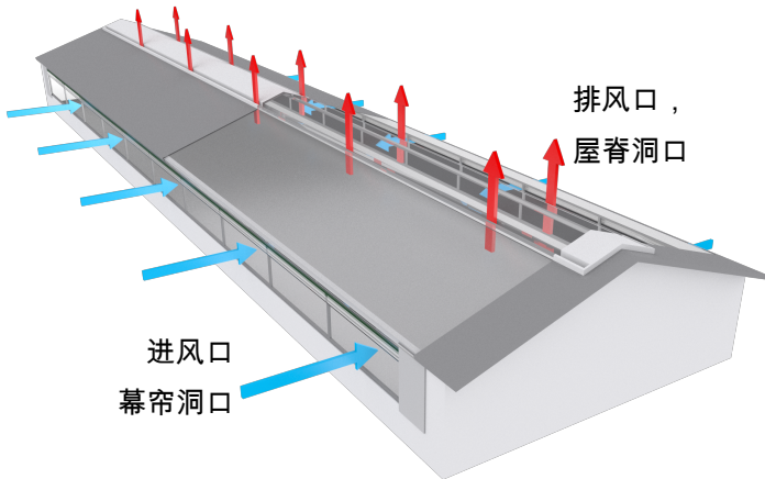
图 18：例如，在通过房屋两侧的幕帘洞口或屋顶的屋脊洞口进行纯自然通风的房舍上。
