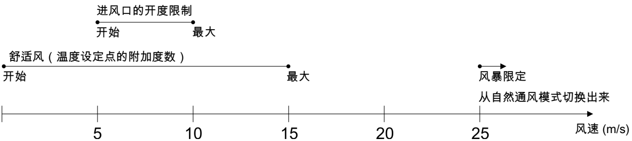
图 23: 风速增加时的自然通风
