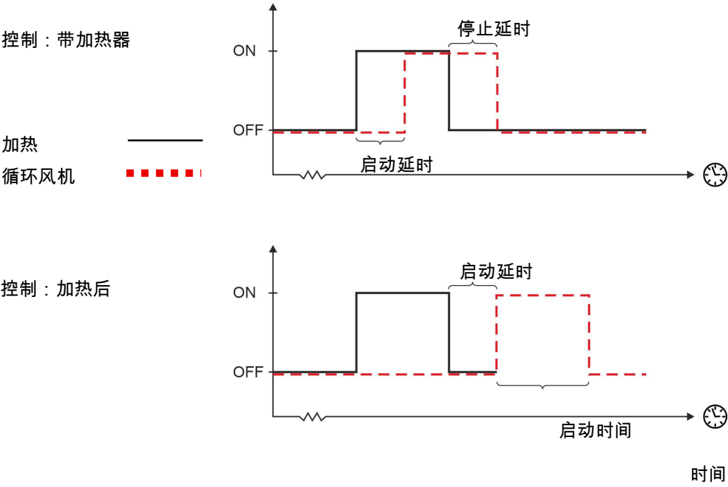
图 25：用加热器控制
